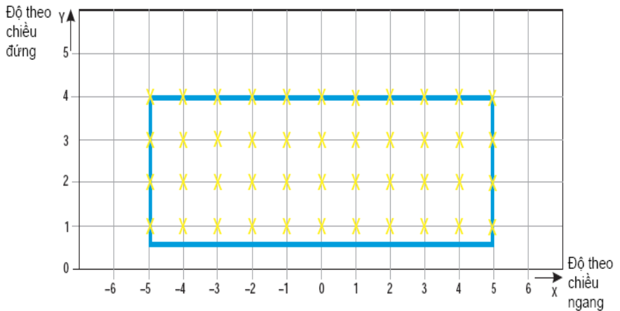
Hình A2-21. Biểu đồ ô vuông đường đẳng sáng sử dụng cho tính toán cường độ trung bình của đèn tìm đường lăn và đèn vạch dừng
