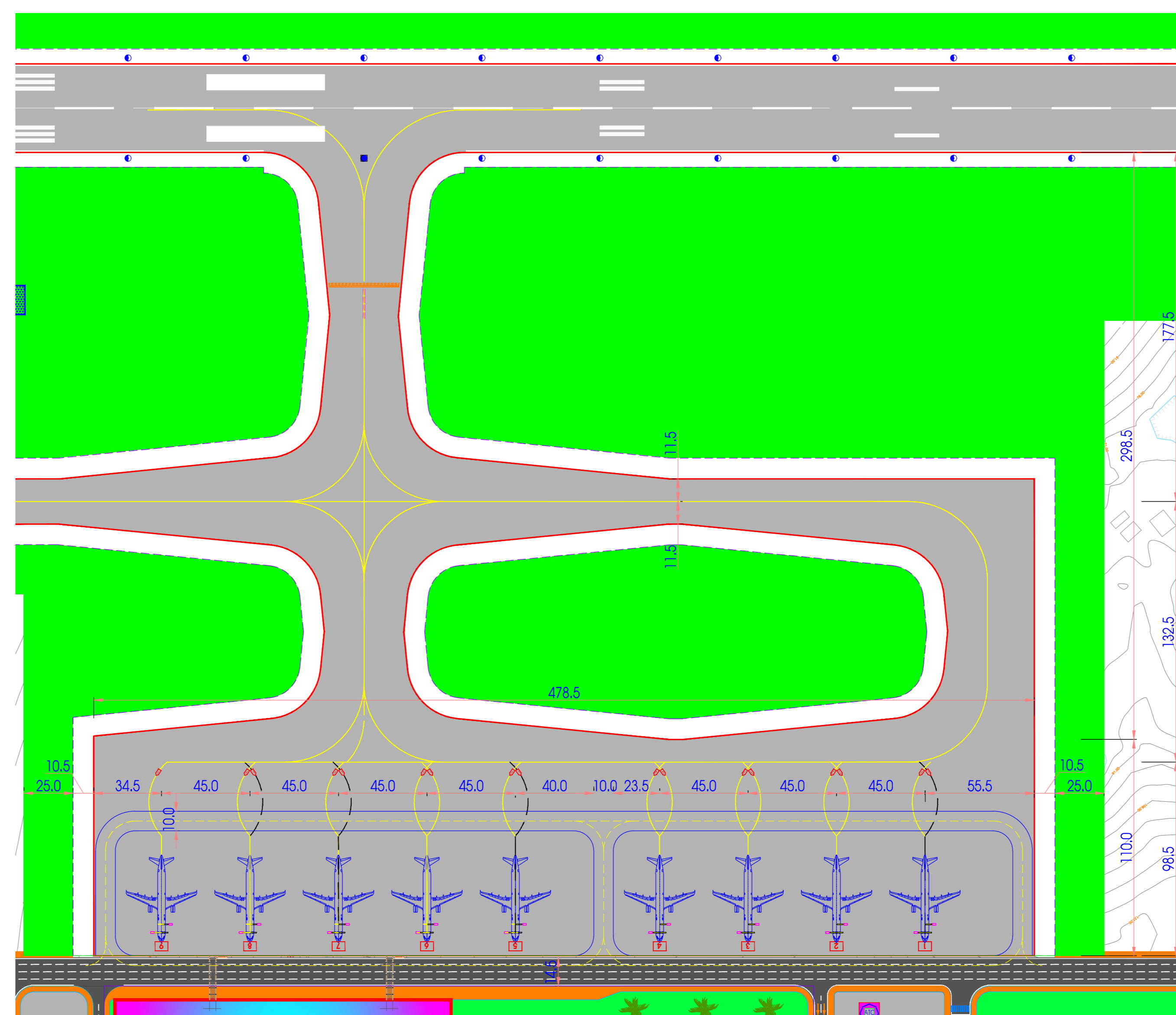
MẶT BẰNG ĐƯỜNG LĂN, SÂN ĐỒ
