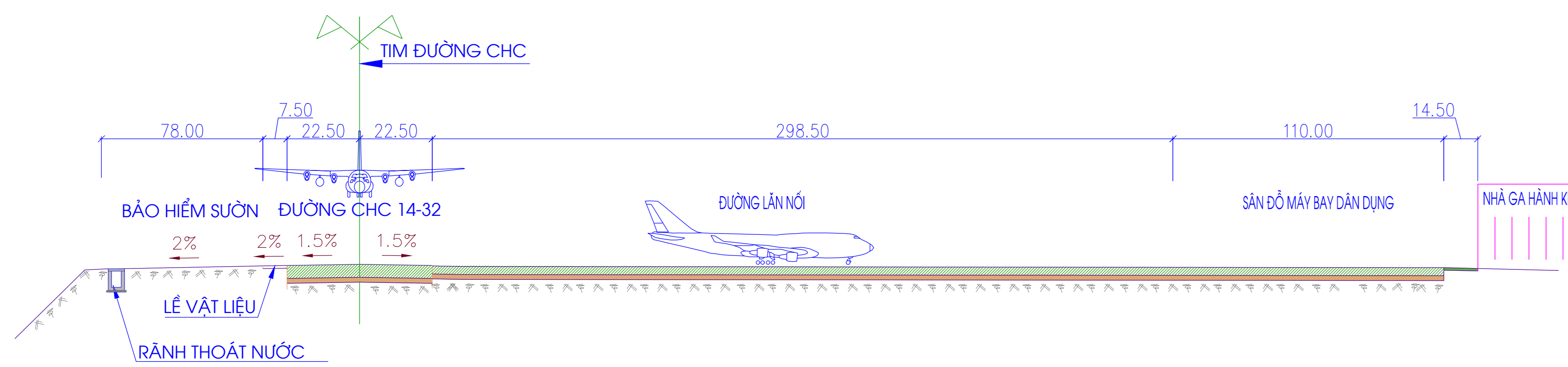
MẶT CẮT 2-2
