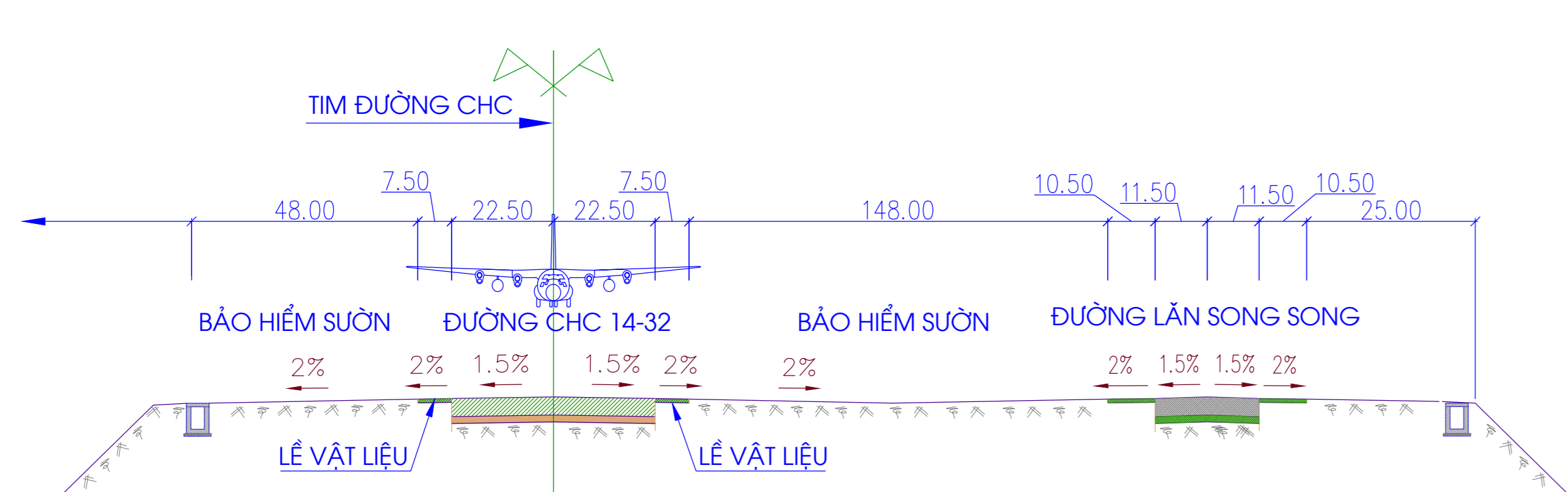
MẶT CẮT 2-2
