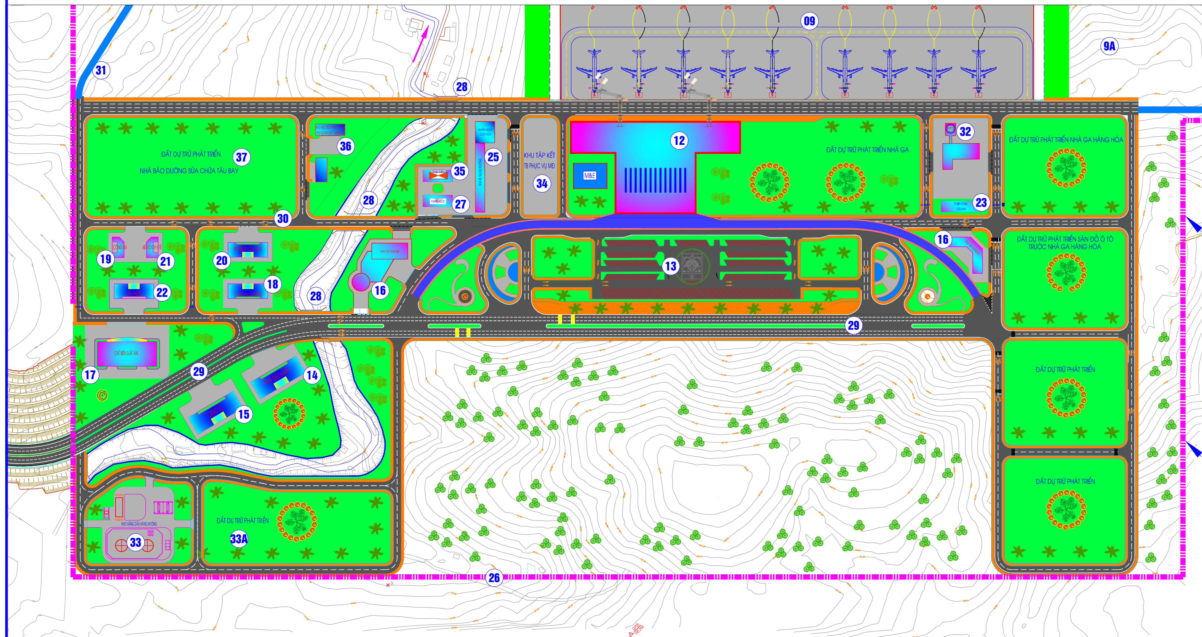
MẶT BẰNG KHU HÀNG KHÔNG DÂN DỤNG
