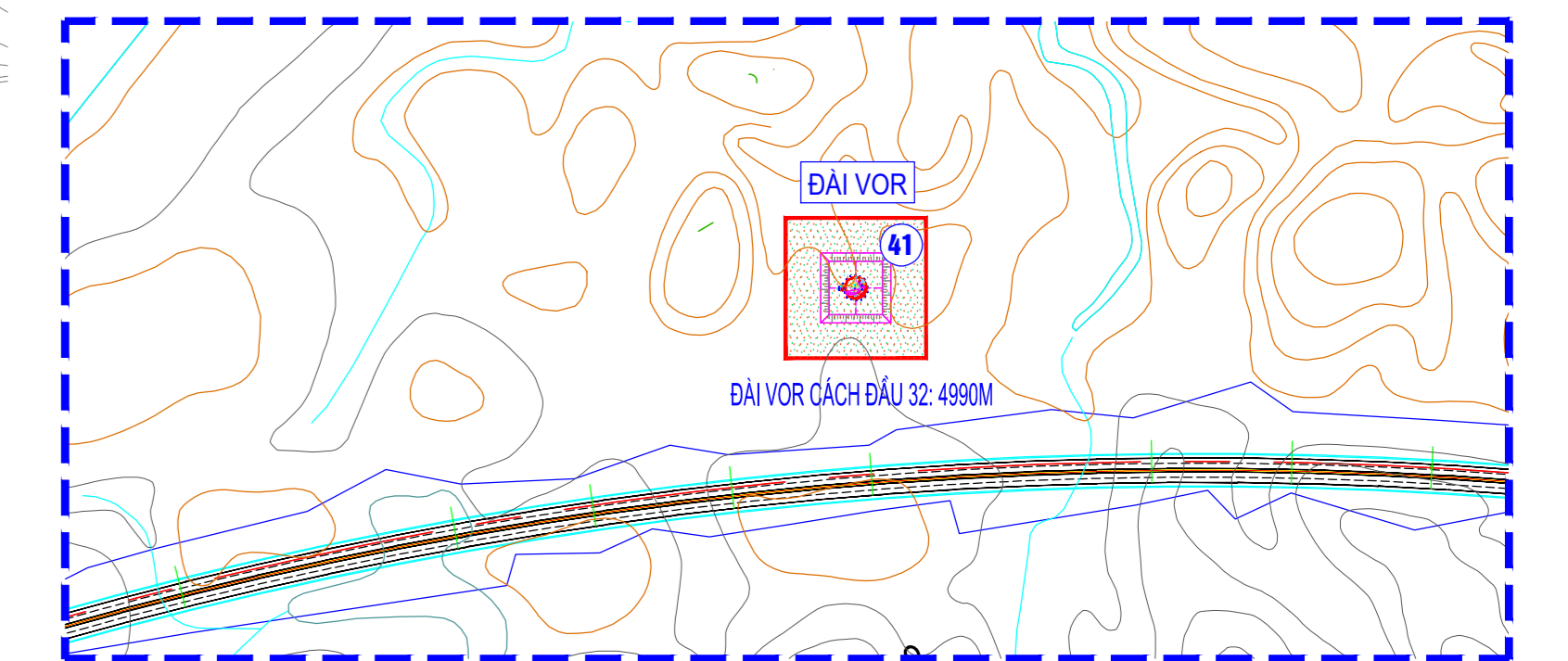
VỊ TRÍ ĐÀI VOR (CÁCH ĐẦU 32 ĐƯỜNG CHK: 4990M)
