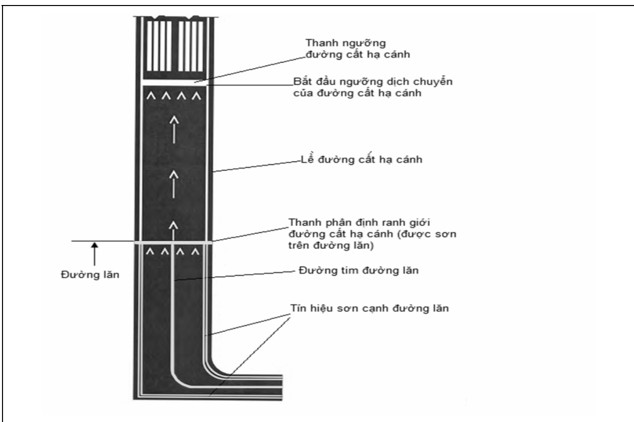
Hình 6. Sơn tín hiệu cho đường lăn kết nối vào đầu ngưỡng đường CHC trước ngưỡng dịch chuyển
