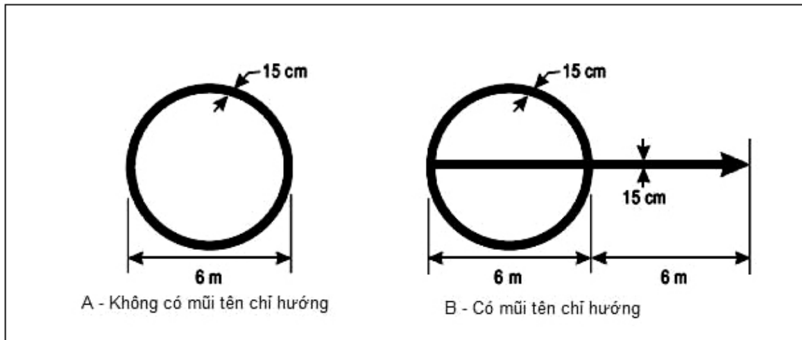
Hình 49. Sơ đồ tín hiệu đánh dấu điểm kiểm tra đài VOR
