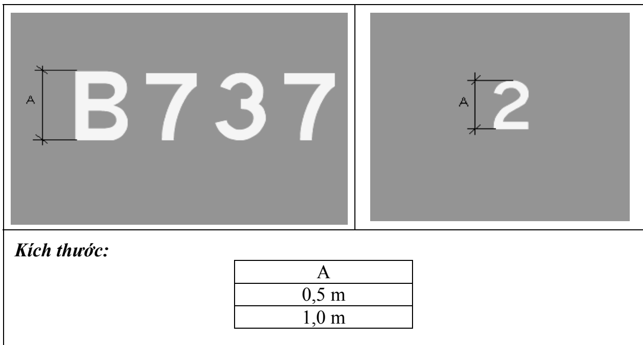
Hình 41. Số hiệu loại tàu bay khai thác
