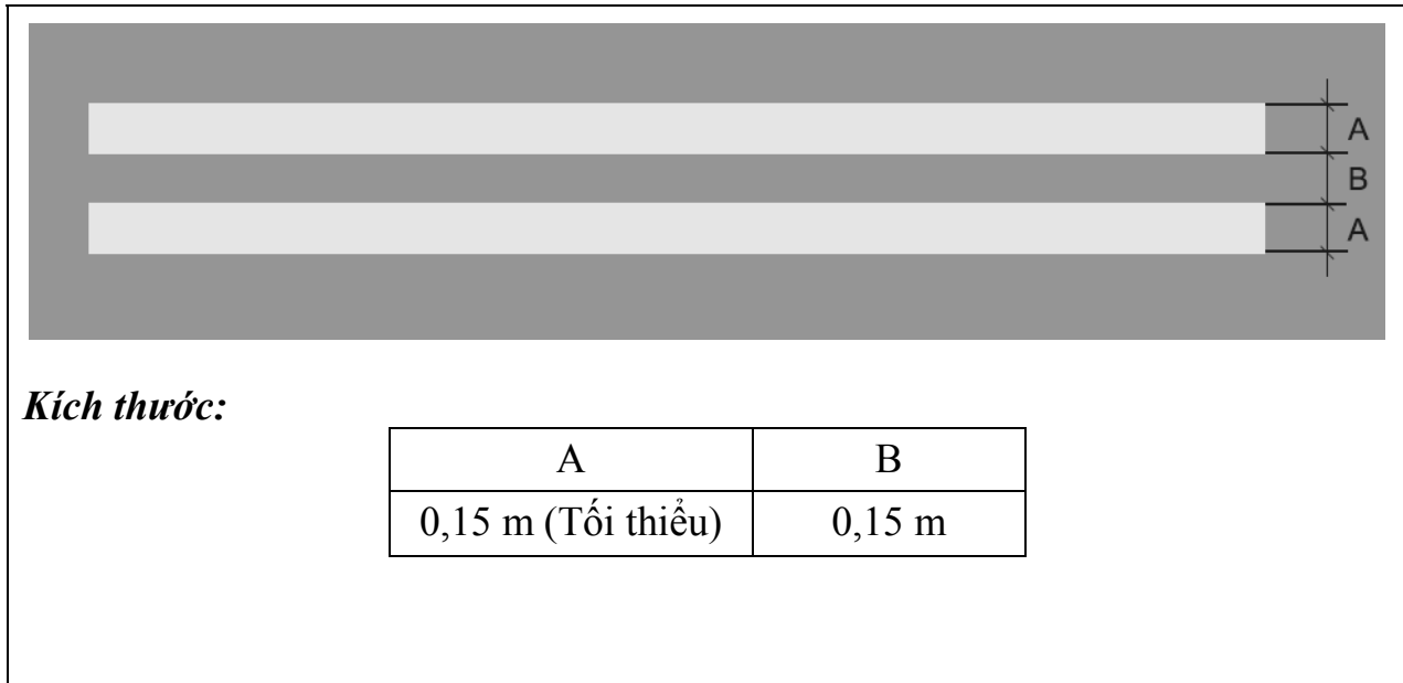
Hình 18. Sơn tín hiệu cạnh đường lăn và sơn tín hiệu đường giới hạn sân đỗ tàu bay
