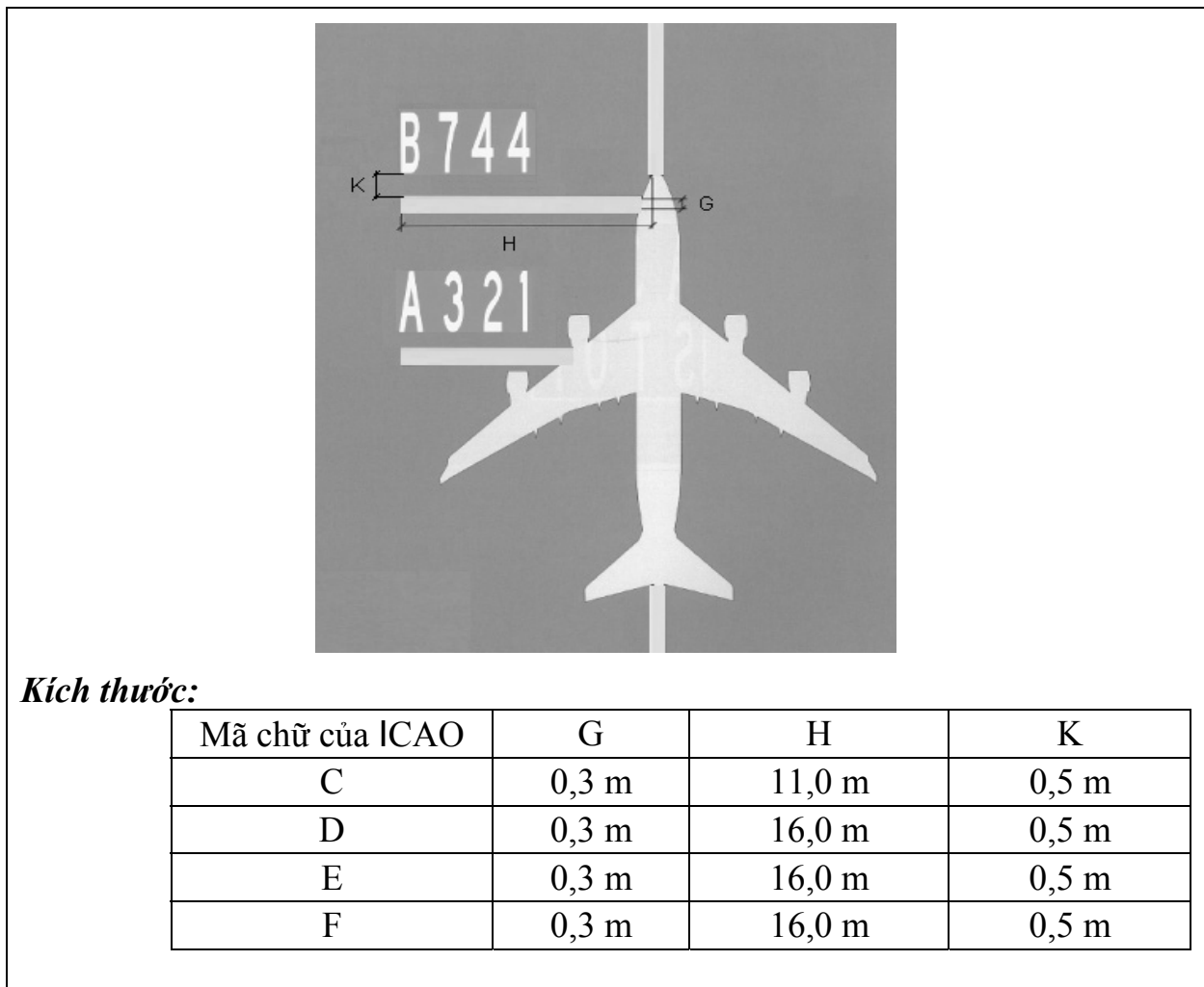
Hình 39. Sơn tín hiệu dừng bánh mũi (nhiều vạch dừng, mỗi một vạch sử dụng tương ứng cho từng loại tàu bay khai thác)
