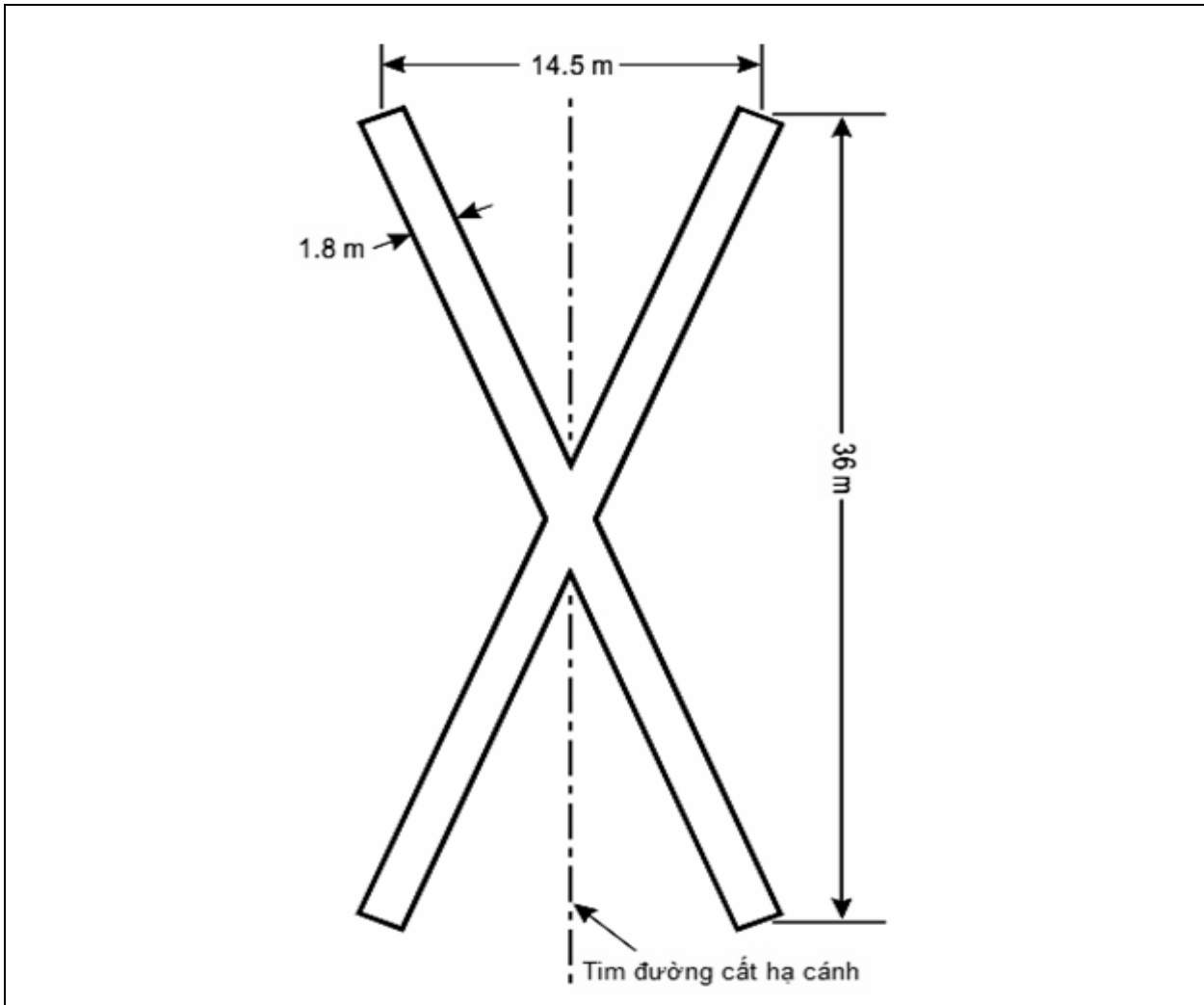
Hình 11. Sơn tín hiệu đóng cửa đường cất hạ cánh
