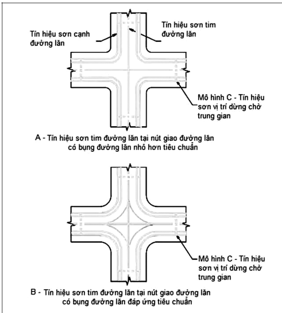
Hình 13. Sơn tín hiệu đường tim đường lãn
