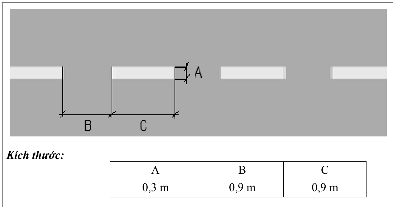
Hình 17. Sơn tín hiệu vị trí chờ lãn trung gian
