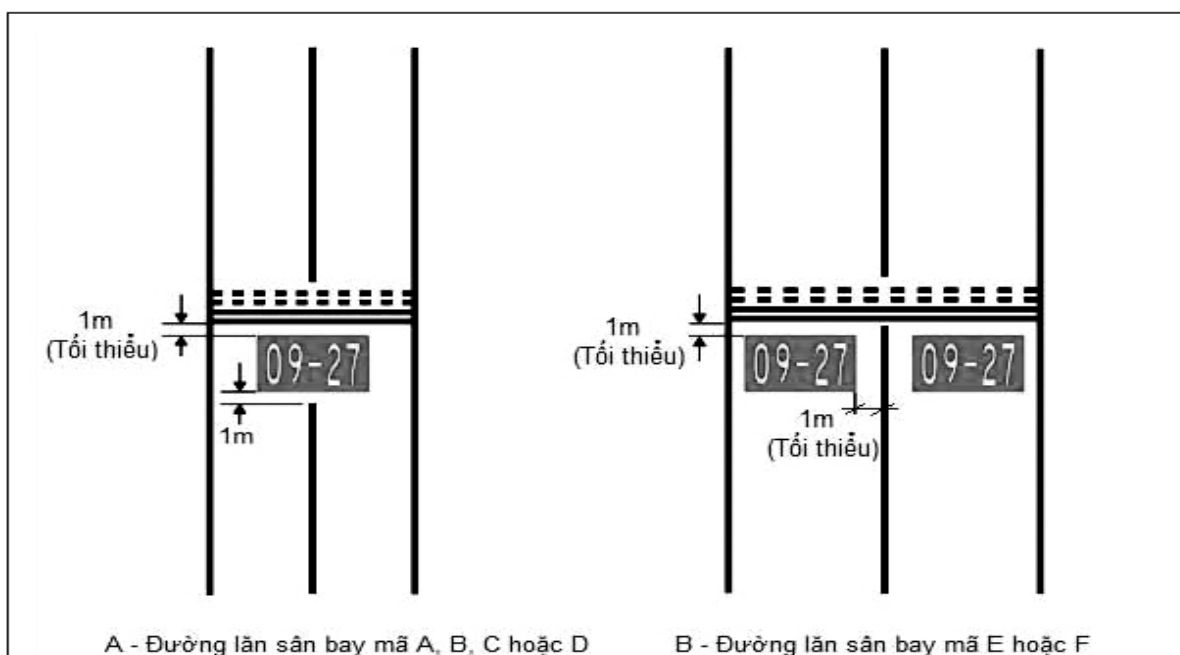
Hình 23. Sơn tín hiệu chỉ dẫn bắt buộc
