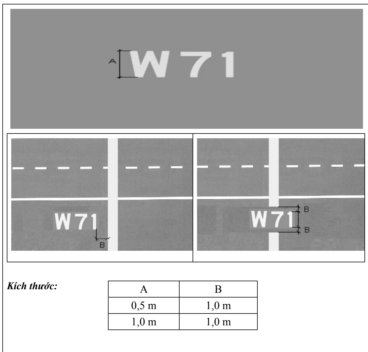
Hình 35. Sơn tín hiệu vị trí đỗ tàu bay
