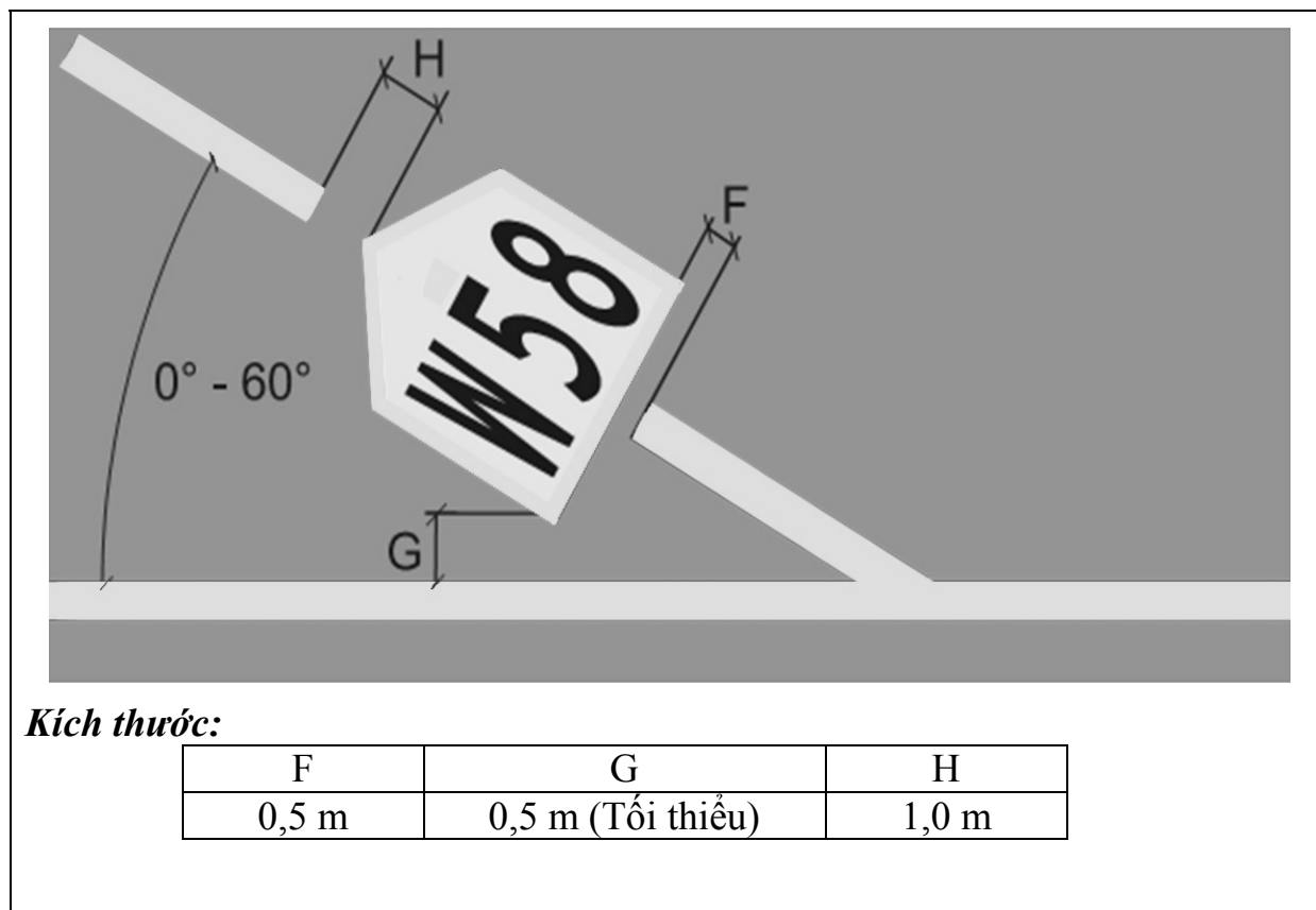
Hình 31. Sơn tín hiệu nhận dạng đến vị trí đỗ tàu bay (Góc 0° đến 60°)
