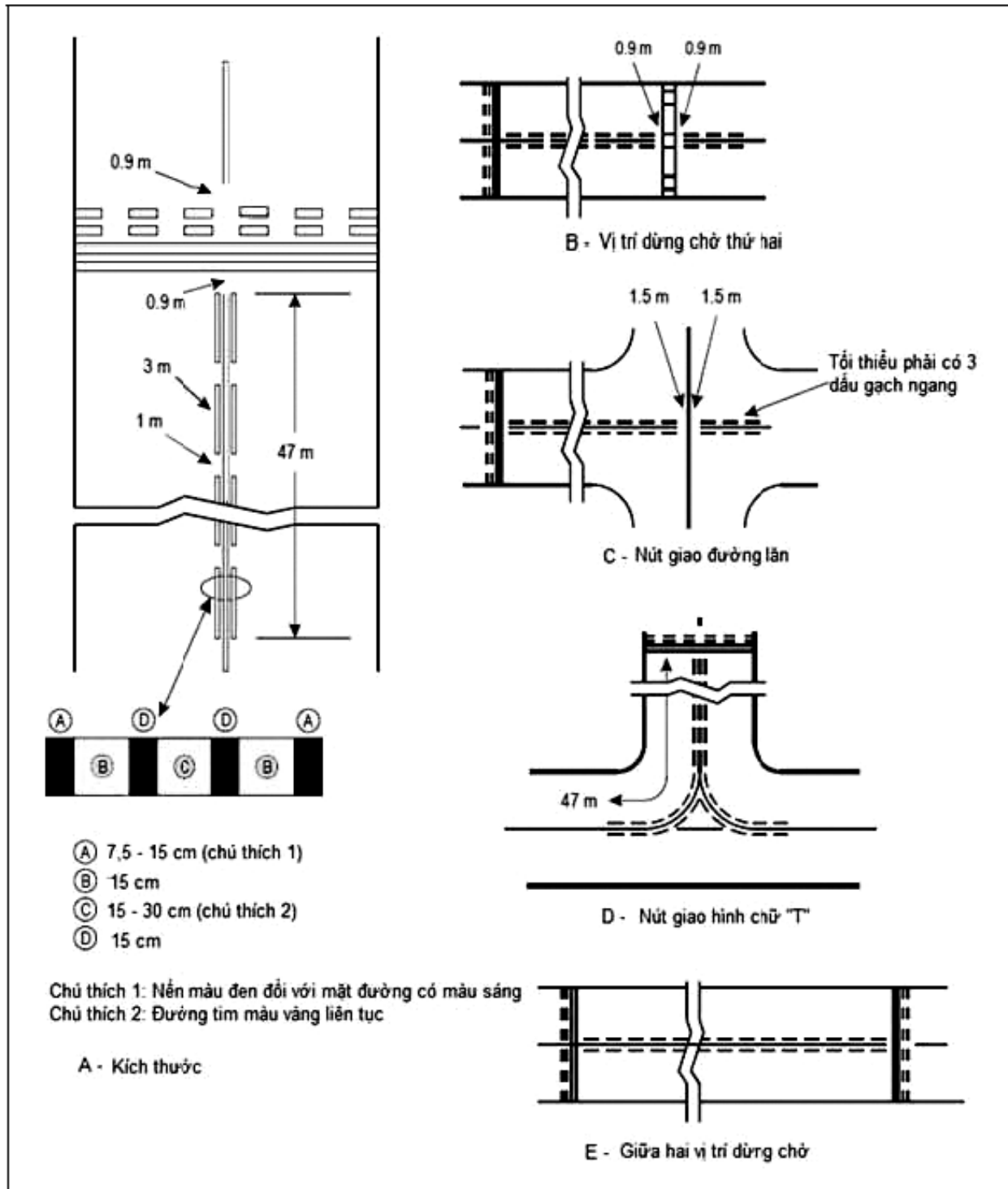
Hình 14. Sơn tín hiệu tăng cường cho đường tim đường lăn
