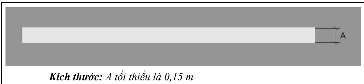
Hình 9. Hình dạng, kích thước của sơn tín hiệu đường tim đường lăn, sơn tín hiệu sân quay đầu đường CHC
