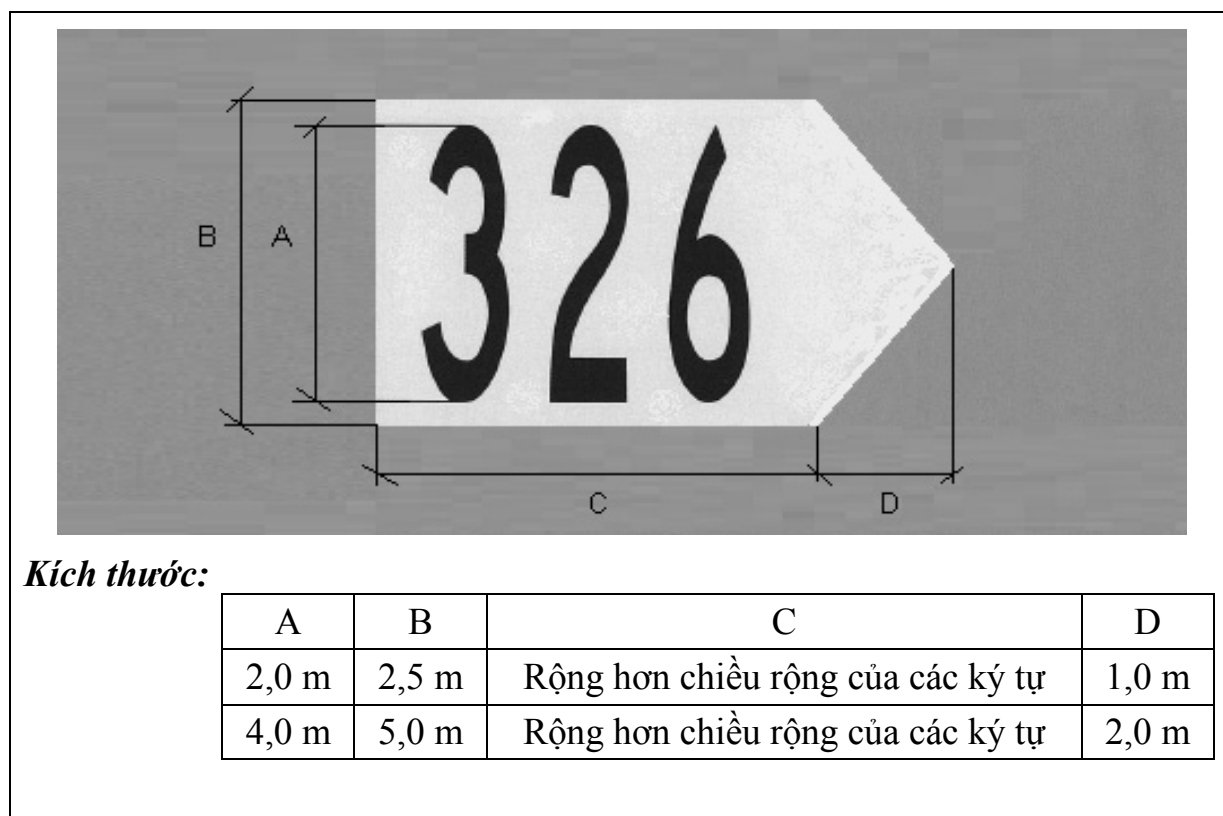
Hình 32. Sơn tín hiệu nhận dạng đến vị trí đỗ tàu bay (Góc 61° đến 90°)
