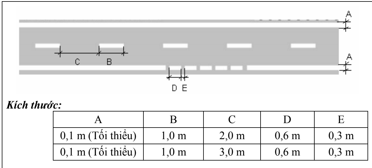
Hình 46. Sơn tín hiệu đường công vụ cho các phương tiện mặt đất
