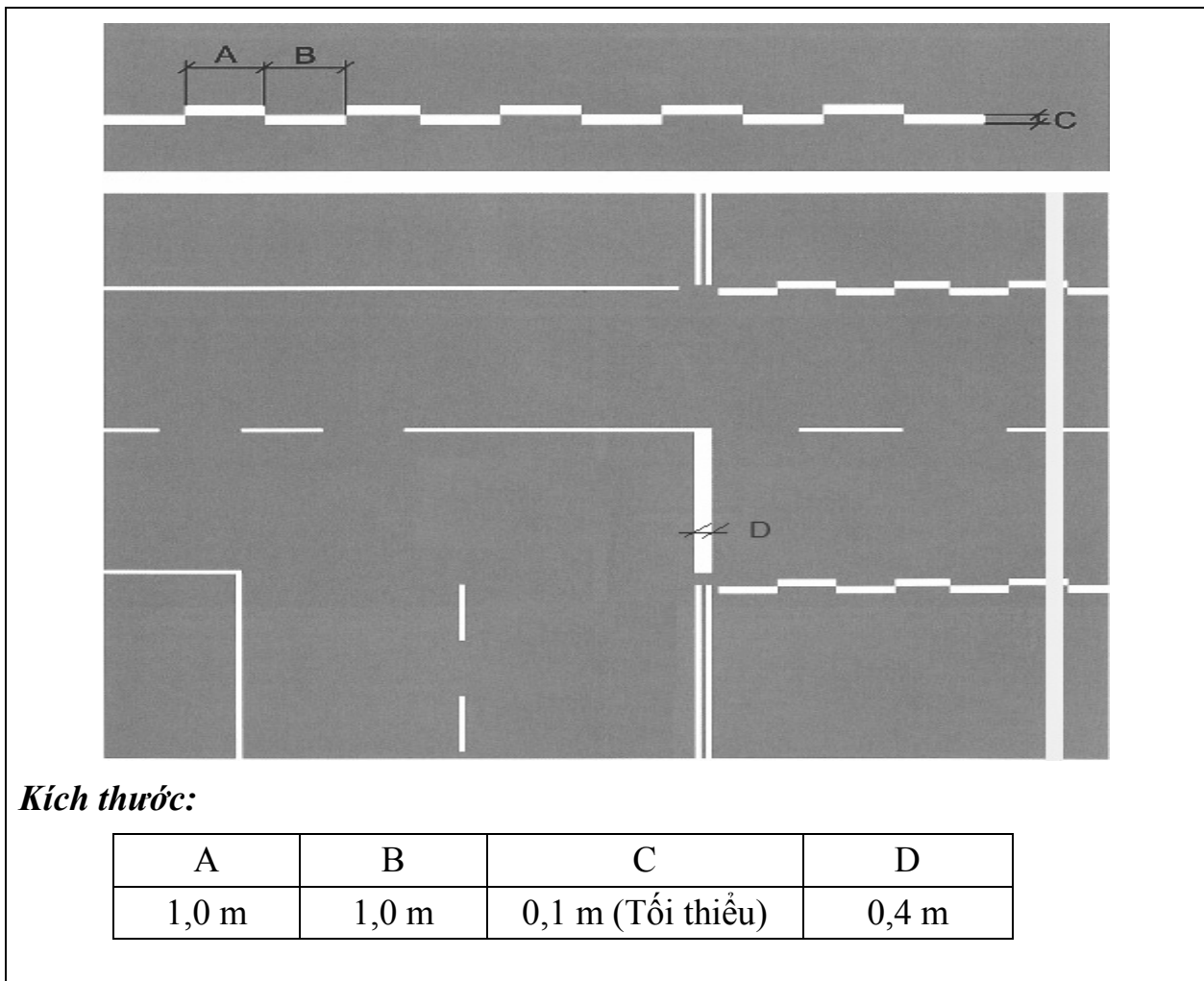
Hình 47. Sơn tín hiệu đường công vụ cho các phương tiện mặt đất cắt ngang qua đường lăn hoặc vệt lăn của tàu bay
