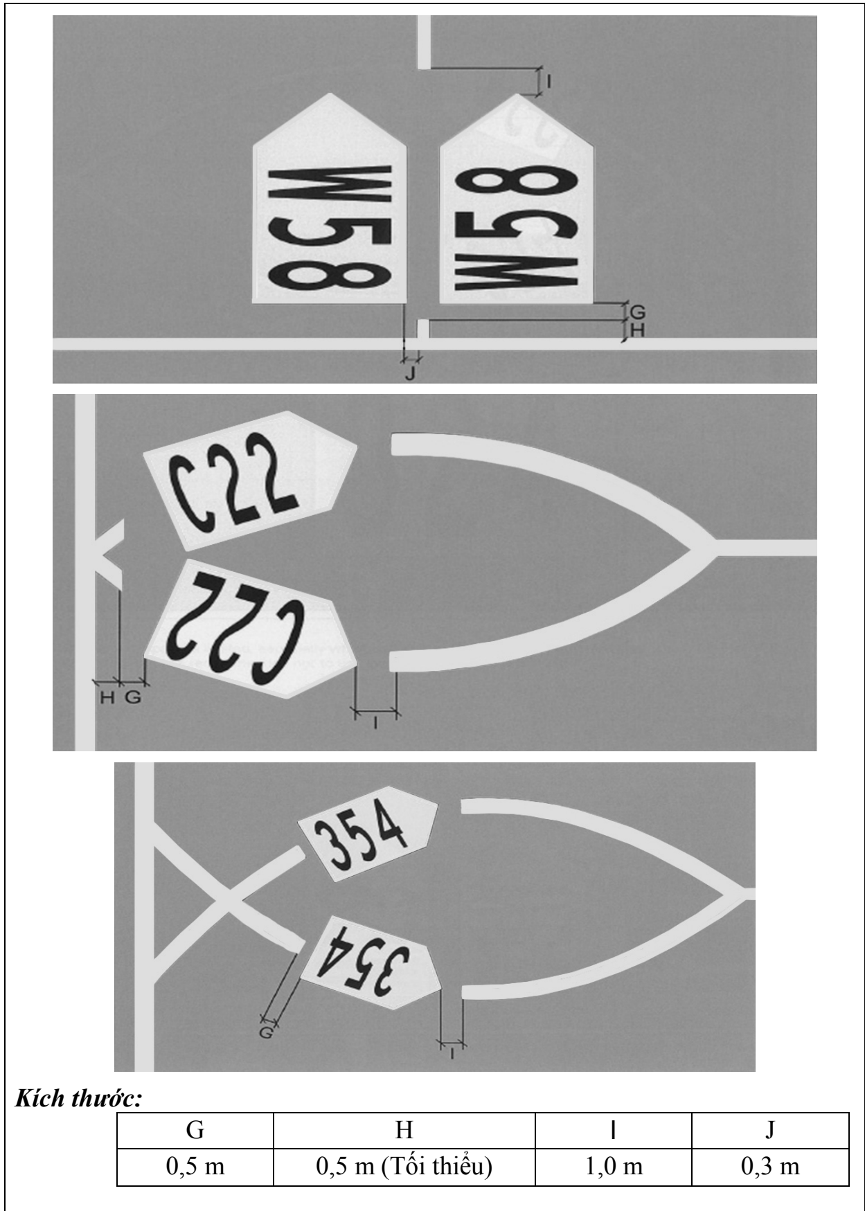
Hình 34. Sơn tín hiệu nhận dạng đến vị trí đỗ tàu bay (Góc 61 0 đến 90 0 )
