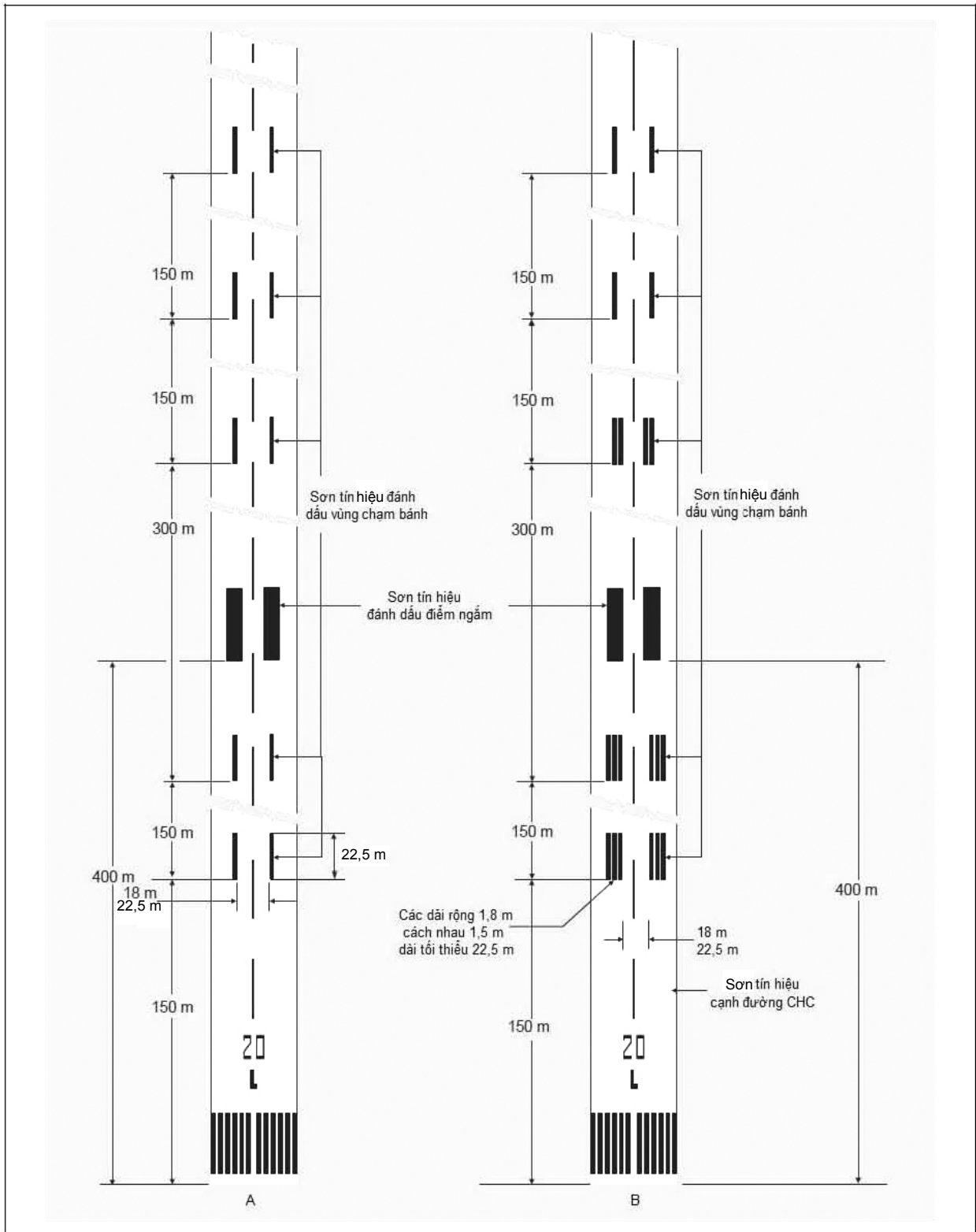
Hình 7. Sơn tín hiệu đánh dấu điểm ngắm và vùng chạm bánh (minh họa cho đường CHC có chiều dài từ 2400 m trở lên)
