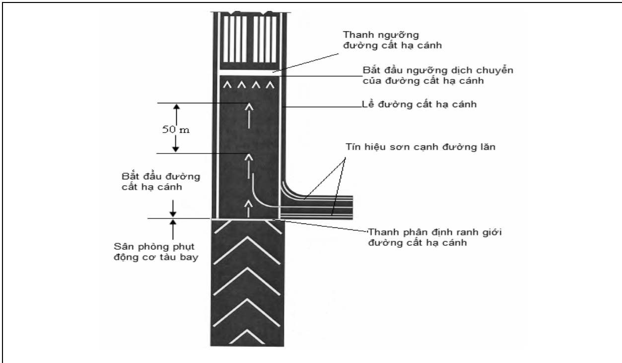
Hình 5. Sơn tín hiệu sân phòng phụt động cơ tàu bay trước ngưỡng dịch chuyển của đường cất hạ cánh
