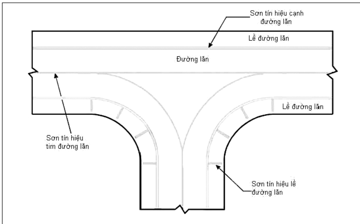
Hình 21. Sơn tín hiệu lề đường lên (Tại nơi đường lên giao với đường lên)
