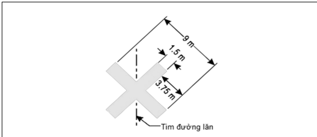
Hình 22. Sơn tín hiệu đóng cửa đường đường lăn
