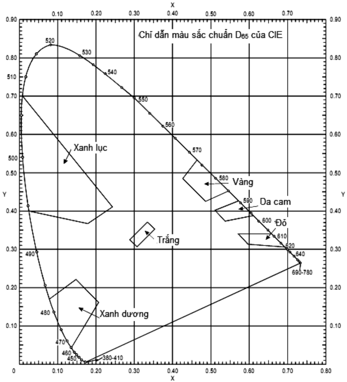
Hình B2. Biểu đồ màu sắc của sơn tín hiệu phản quang
