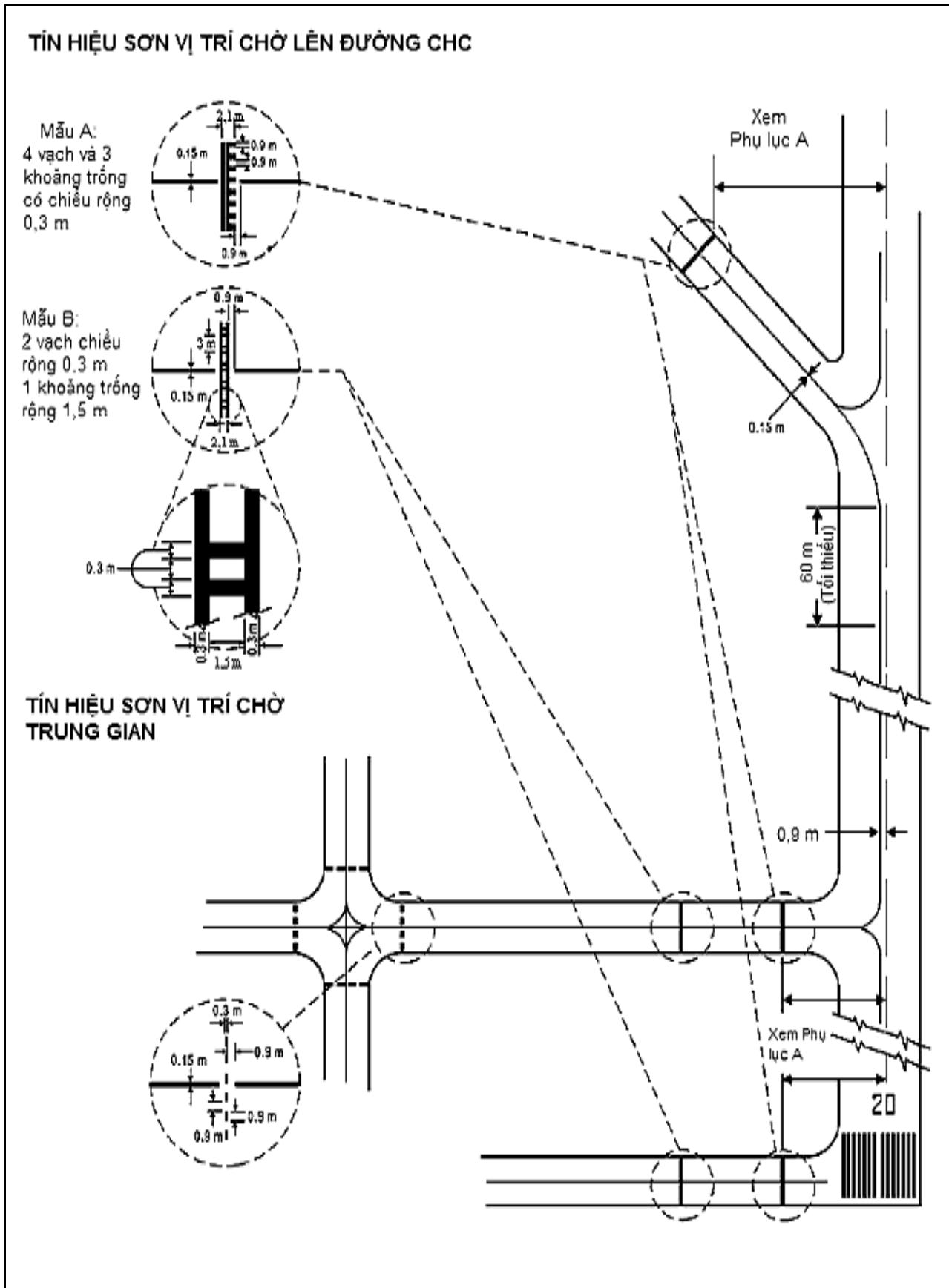
Hình 12. Sơn tín hiệu đường lãn
