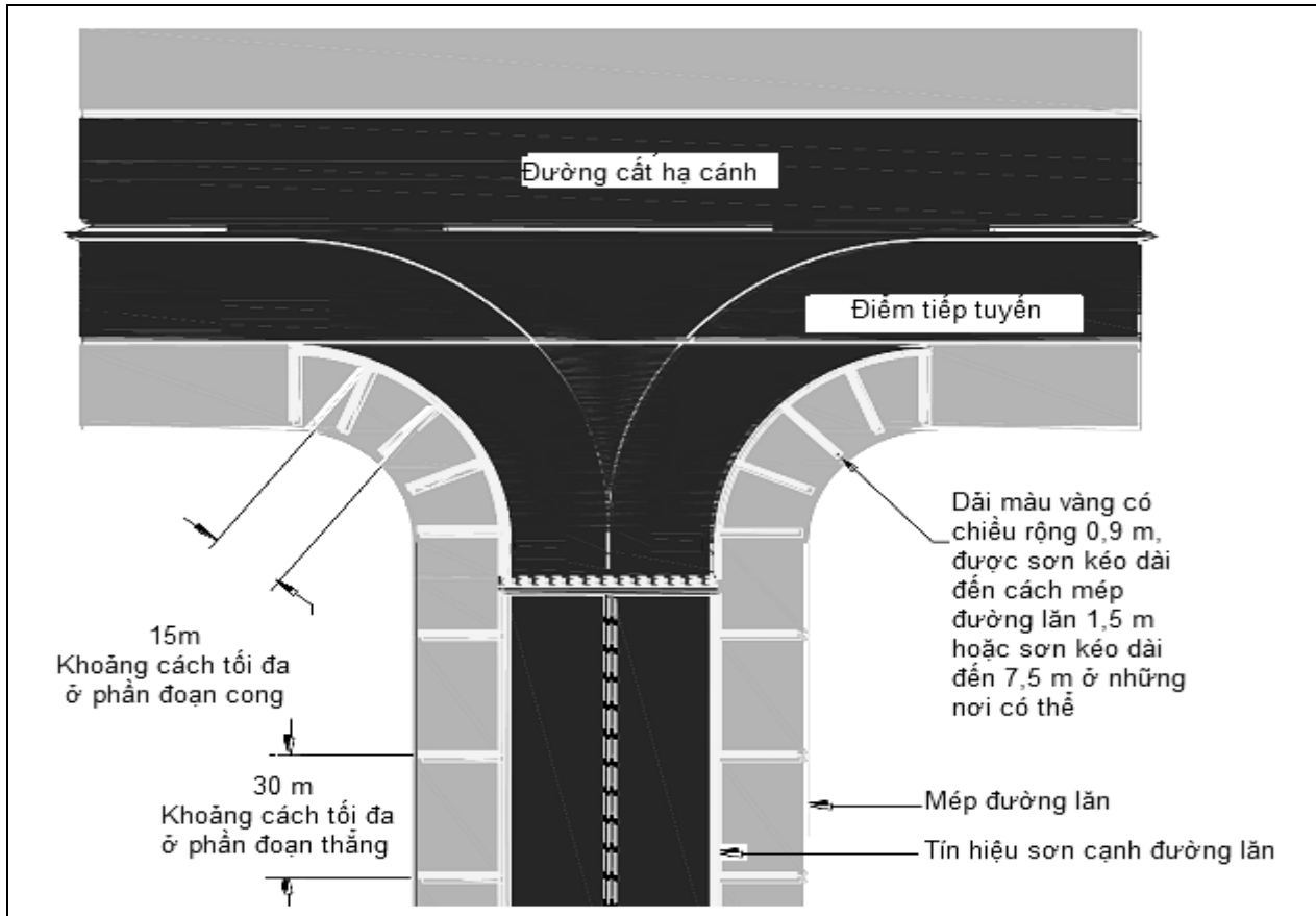
Hình 20. Sơn tín hiệu lề đường lên (Tại nơi đường lên giao với đường CHC)
