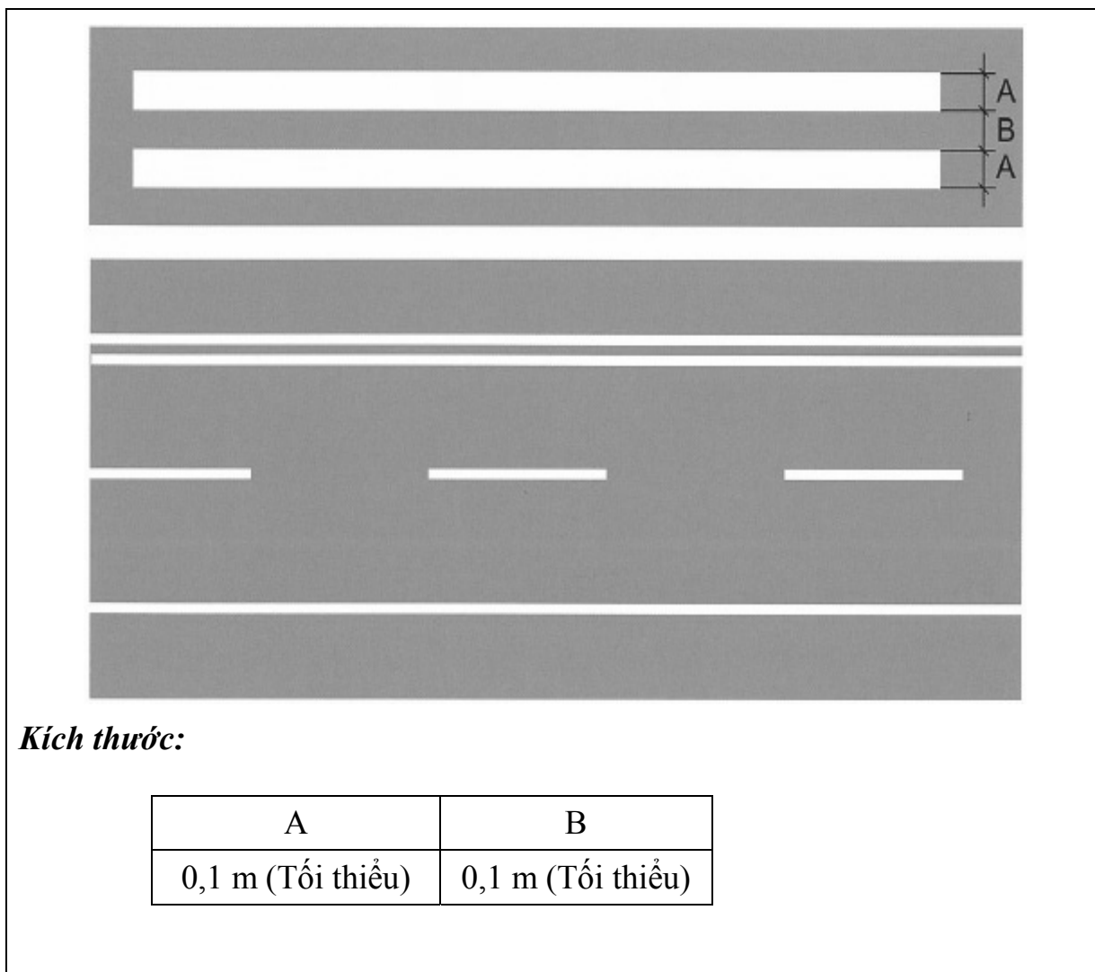
Hình 48. Sơn tín hiệu giới hạn phương tiện
