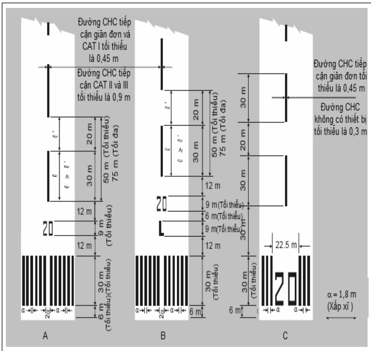
Hình 1. Sơn tín hiệu chỉ hướng đường cất hạ cánh, đường tim và ngưỡng đường cất hạ cánh
